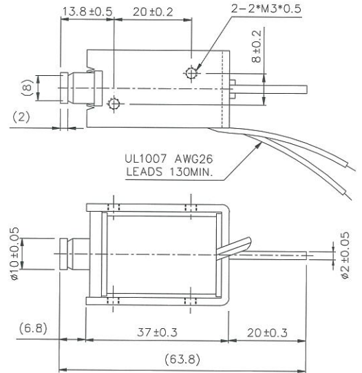
Shown Energized 通電狀態 UNIT 單位 : mm
