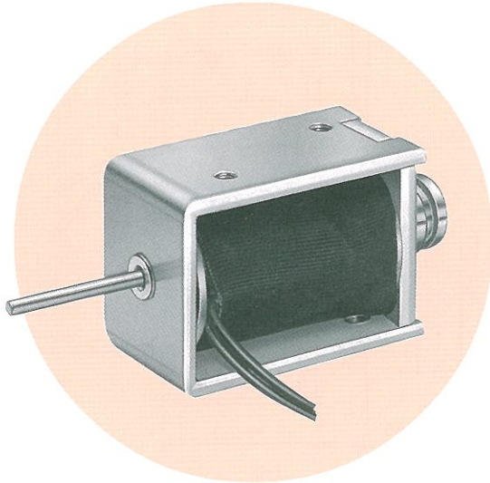
Plunger Weight 可動鐵心重量 : 19g Total Weight 總重量 : 96g
